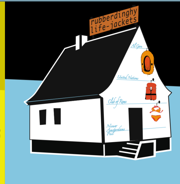
'Sea Level'
